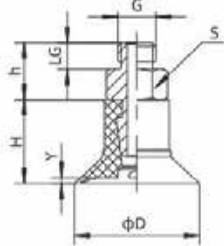
SZF15□-M5M 外螺纹连接
