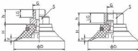
SZF40-50 外螺纹连接
