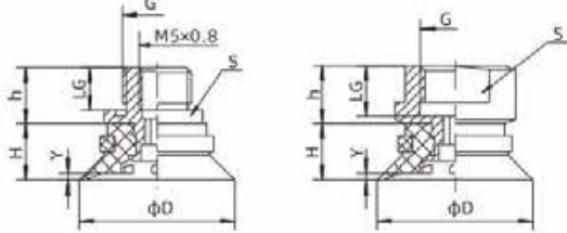
SZF20-30 外螺纹连接
