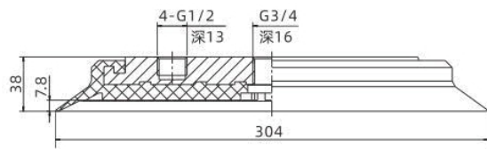
SZF300 内螺纹连接
